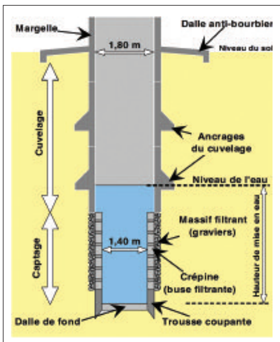
Figure 5 - Schéma de puits moderne (source PSEAU ( https://www.pseau.org/fr document développer les services de l'eau potable 18 questions pour agir)
